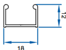
Coupe rail latéral 2 voies
