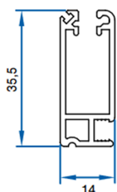
Coupe profil de cadre
