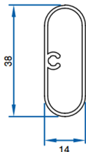
Coupe profil de renfort
