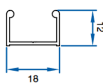
Coupe rail bas 2 voies
