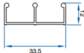
Coupe rail haut 3 voies
