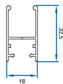
Coupe rail bas 2 voies
