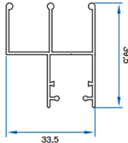
Coupe rail haut 3 voies
