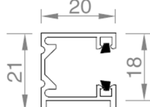
Coulisse renforcée
