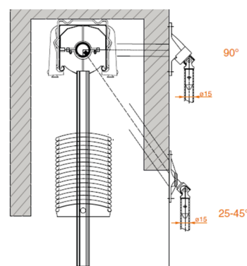
Coupe de principe commande par manivelle
