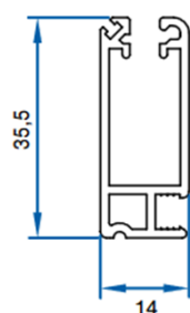
Coupe profil de cadre
