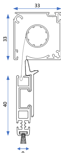
Coupe du boîtier avec tube, toile et barre de charge
