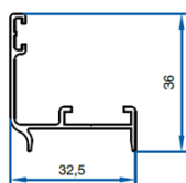
Coupe du dormant
