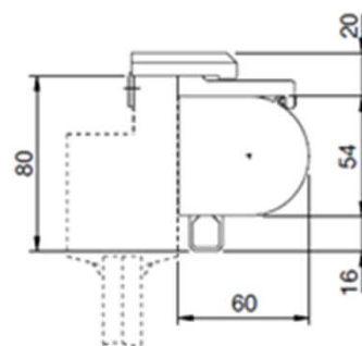
Coupe de principe montage sur le vantail de la fenêtre avec supports sans perçage (option)
