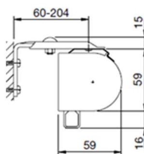
Coupe de principe pose de face Equerres réglables de déport (option)
