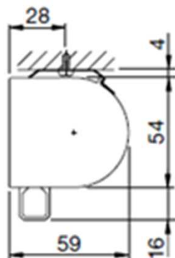
Coupe de principe pose plafond
