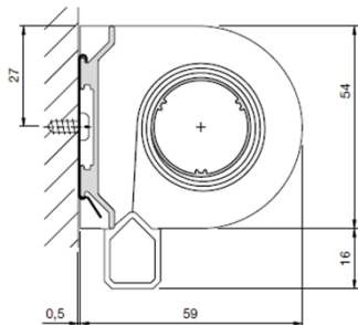
Coupe de principe pose de face
