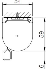
Coupe de principe pose plafond
