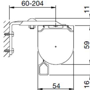
Coupe de principe pose de face Equerres réglables de déport (option)
