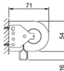
Coupe de principe pose de face Equerres réglables de déport (option)
