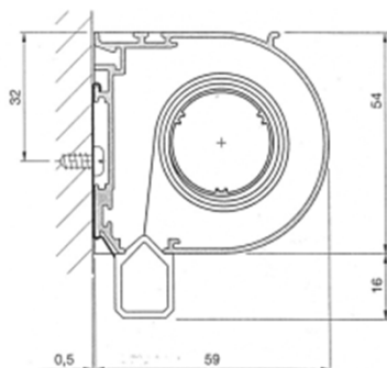
Guidage par câbles gainés noir Schémas de principe
