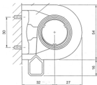
Coupe de principe pose de face
