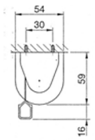
Coupe de principe pose de face Equerres réglables de déport (option)
